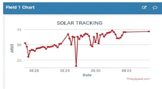
Gambar 4 Grafik output arus pada ThingSpeak.
