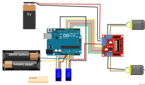
Gambar 4 Prancangan Sistem Elektrik Line Follower
