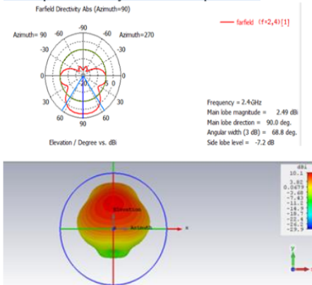
Gbr 7 Pola Radiasi pada Software CST Microwave Studio
