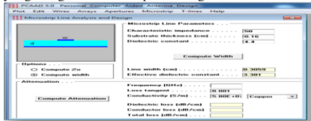
Gbr 2. Perhitungan lebar pencatu dengan menggunakan PCAAD 5.0
