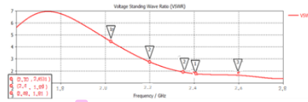
Gbr 6. Nilai VSWR pada CST Microwave Studio
