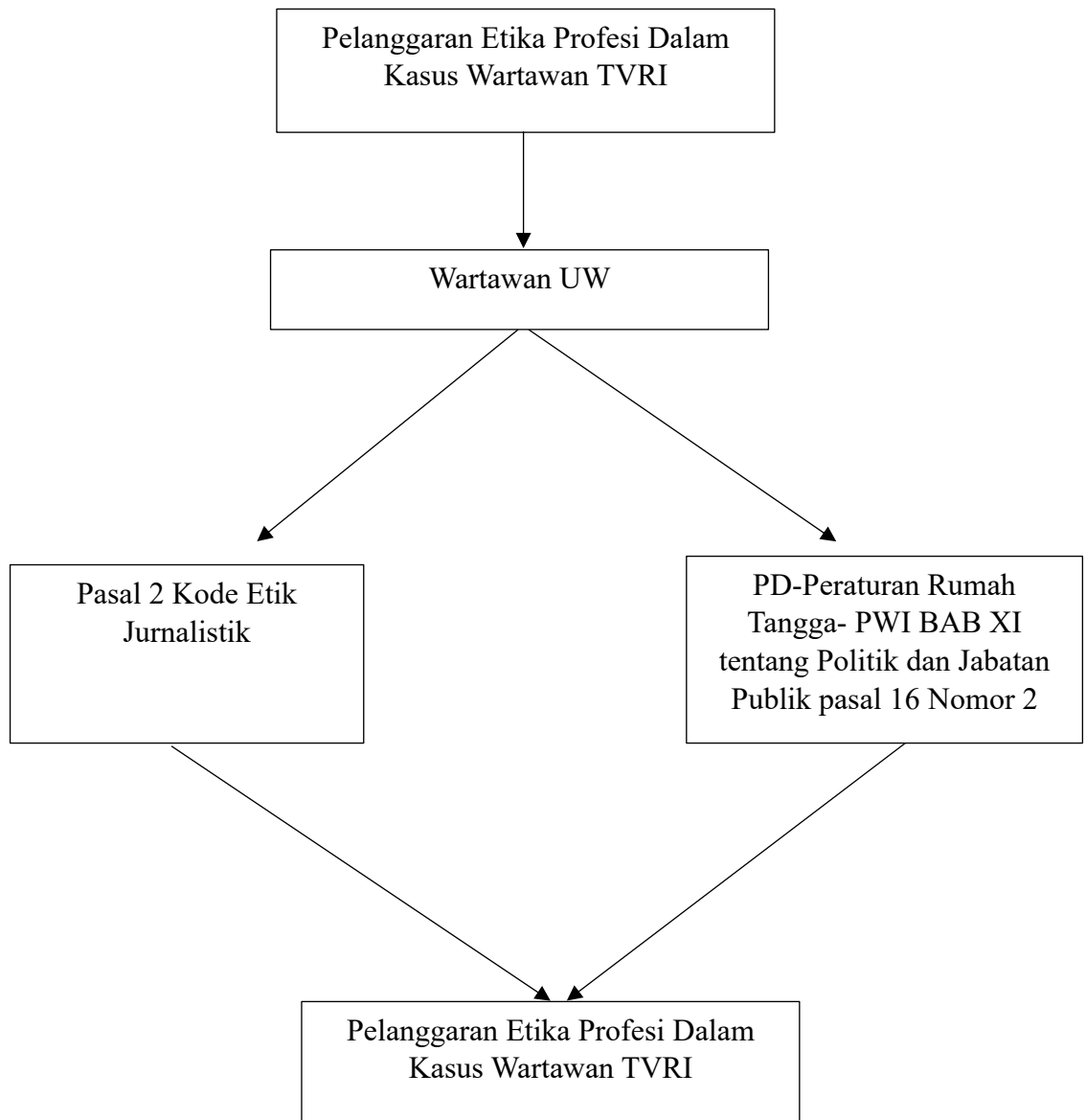
Gambar 2. 1 Kerangka Berpikir
